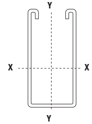
B-902 1½" x 3" x 12 ga. steel
