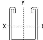
B-901 1¼" x 1½" x 12 ga. steel
