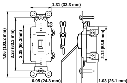
LOCKING 1201-2L, 1221-2L
