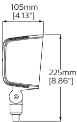
PFL20 Side
