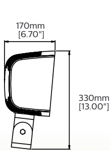
PFL150 Side
