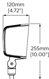
PFL40 Side
