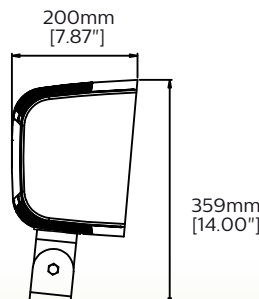
PFL300 Side
