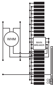
TSM2020CSCU, TSM2020CFCU
