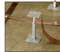
Low Impedance Riser (LIR)
