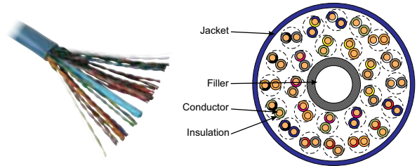
Cat5e 25 Pair
