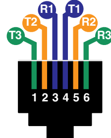
USOC RJ25
