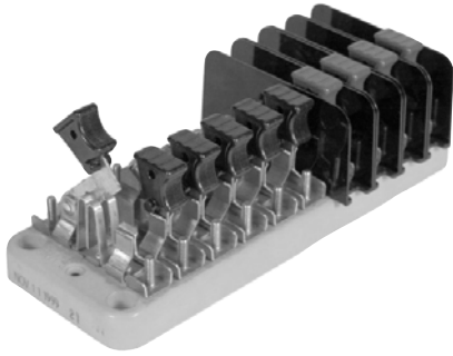
SWITCH BLADES
