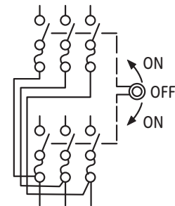
Fusible / 3 Pole / 3 Wire / 240 V
