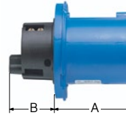
125A Inlet
