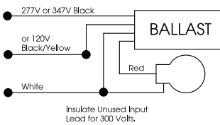
Wiring Diagram 20
