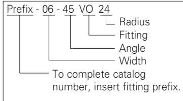
45° (VO) Mitered
