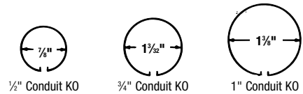
1/2" Conduit KO
