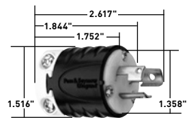
15A Plug
