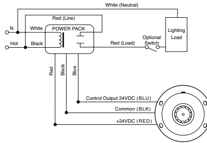
DT300 Wiring
