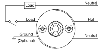
DT355 Wiring
