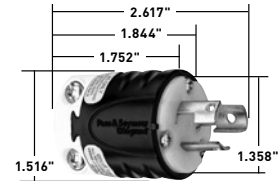
15A Plug
