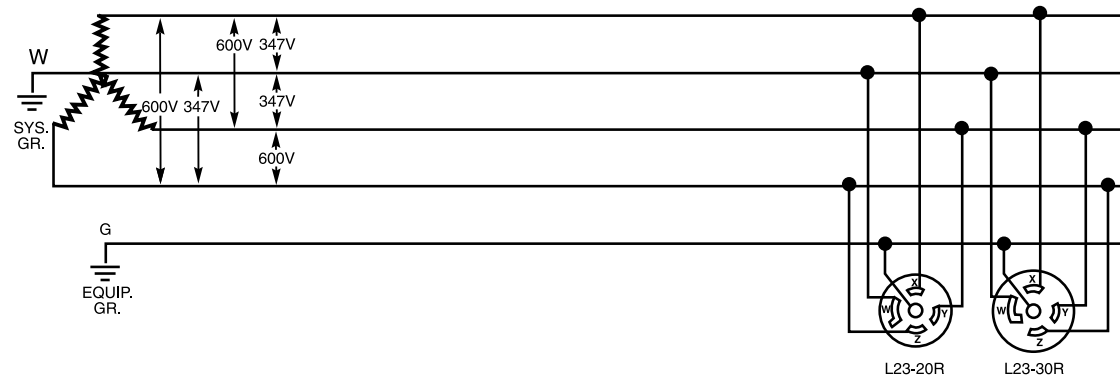
3 \phi Y347/600V
