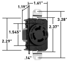
20A Receptacle
