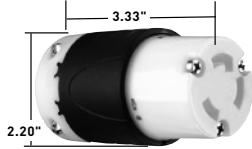
20A Connector
