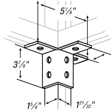
CAT. NO. A218
