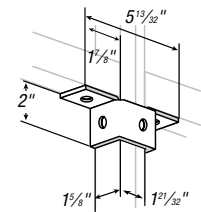
CAT. NO. AW220
