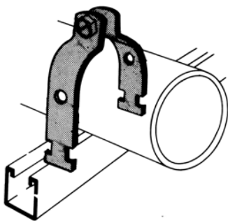
702_AL Rigid Conduit Pipe Strap
