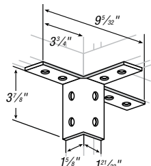
CAT. NO. AW228
