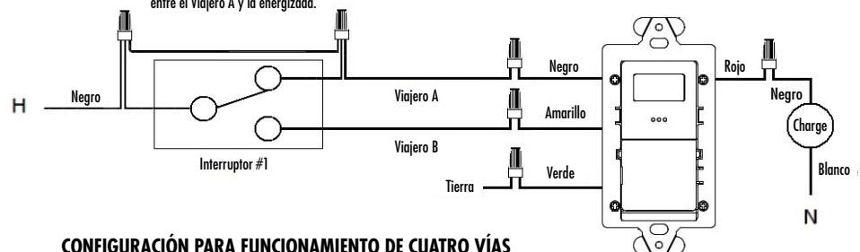
Figura 1 Conecte un conductor dentro de la caja, entre el Viajero A y la energizada.
