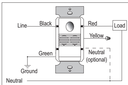
DSW-301 and DSW-301-347 Wiring
