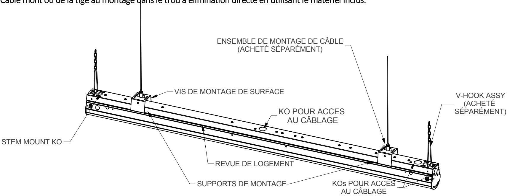
FIG 1 CONFIGURATION AUTONOME
