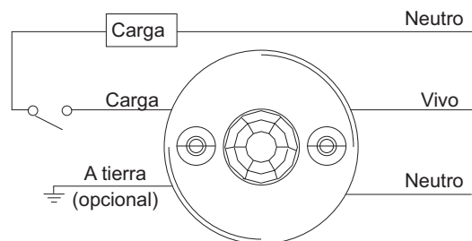
Un sensor, una carga
