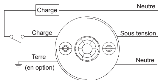
Détecteur seul, charge seule
