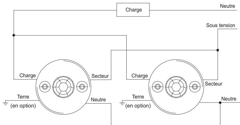
Plusieurs détecteurs connectés en parallèle
