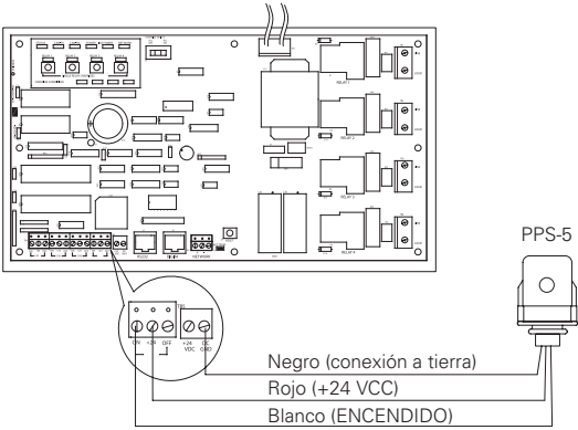
Figura 5. Conexión del ControlKeeper 4
