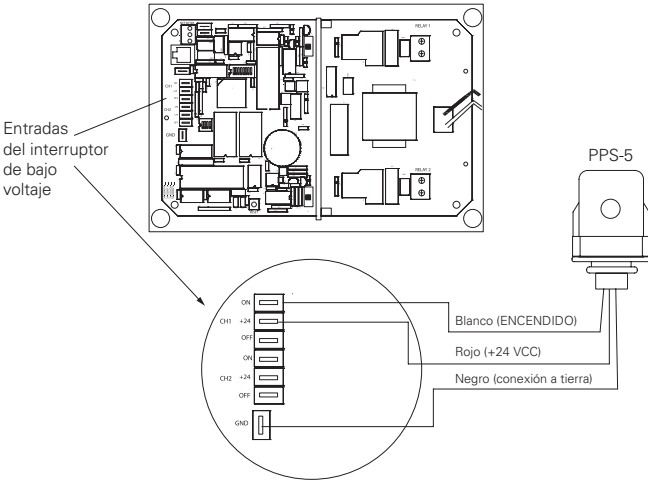
Figura 7. Conexión del ControlKeeper 2
