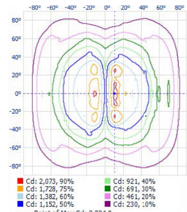
Isofootcandle Plot
