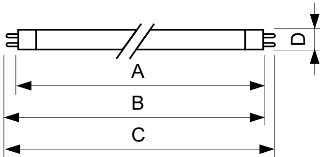
TL5 HO EcoPlus 44=54W/840
