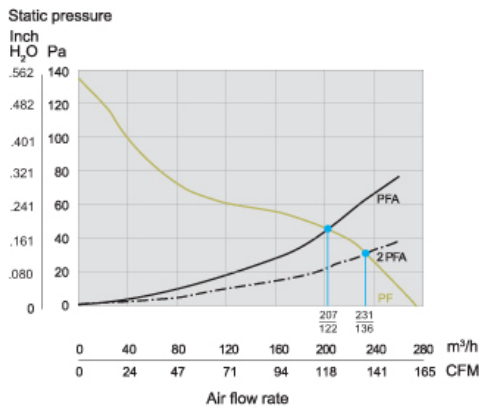
PF 43.000 IP55 / PFA 40.000 IP55
