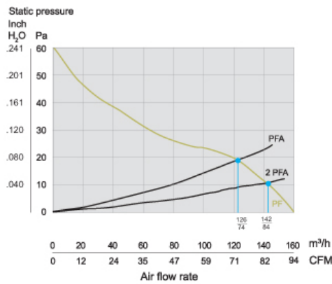
Airflow Data: PF 42.500 IP55 / PFA 40.000 IP55
