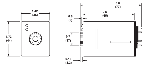
OND-DFSB (DPDT)
