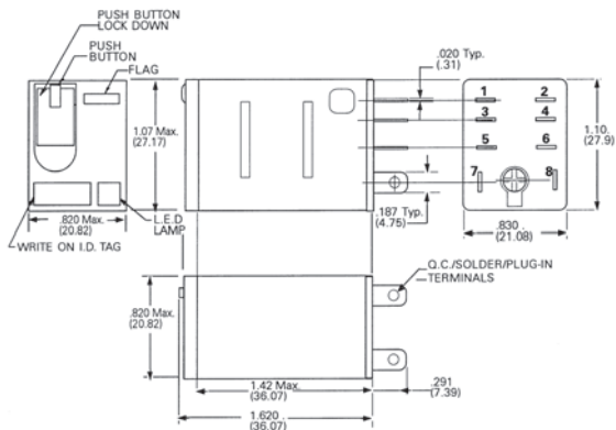
3TX7114 DPDT
