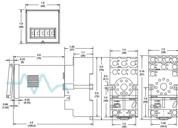
OFD-DFPR-00 (DPDT)
