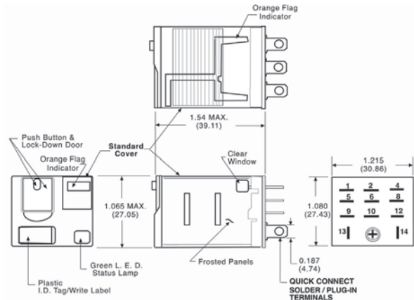
3TX7116 3PDT
