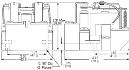
3TX7130 DPDT
