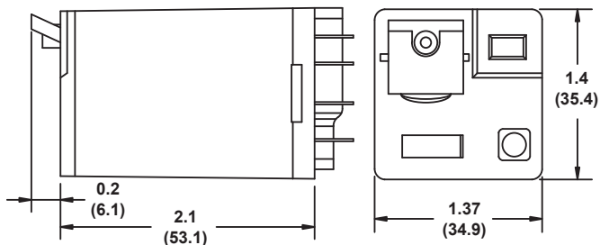
3TX7115 3PDT
