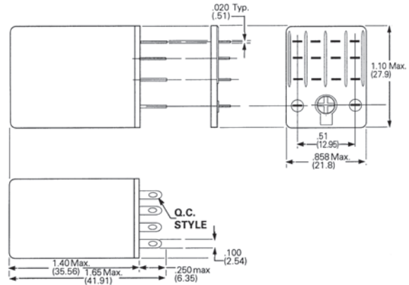
3TX7126
