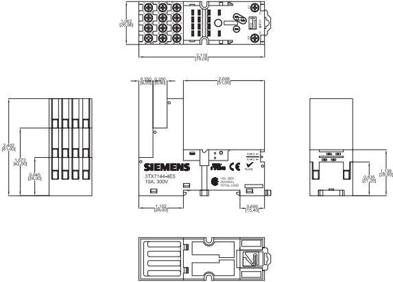
3TX7144-4E5
