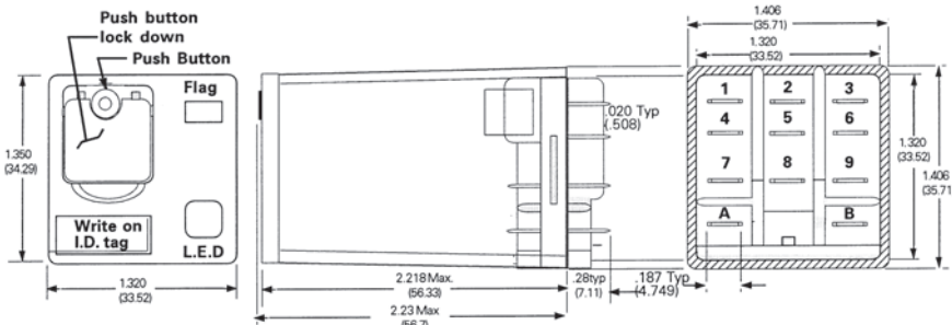
3TX7115 3PDT
