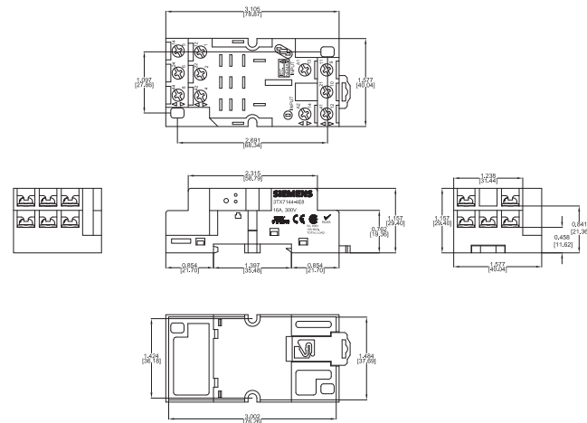
3TX7144-4E8
