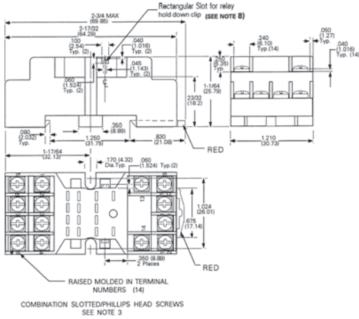
3TX7144-1E7
