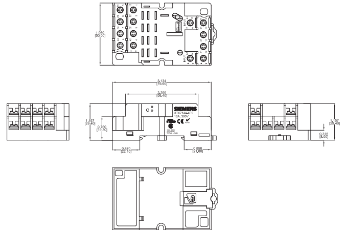
3TX7144-4E9
