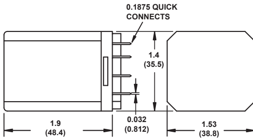
3TX7137 (DPDT)
