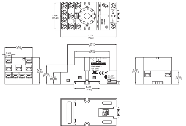
3TX7144-4E3
