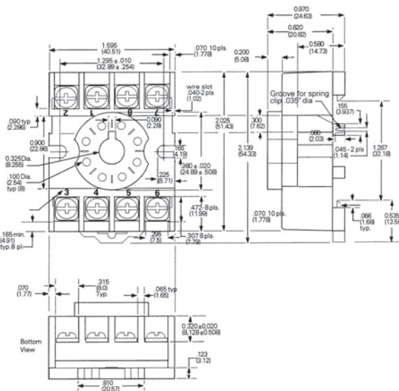
3TX7144-1E2
