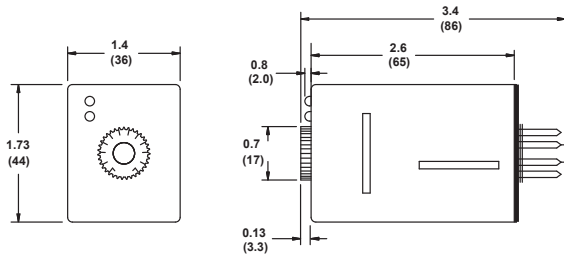
OFD-DFOB (DPDT)
