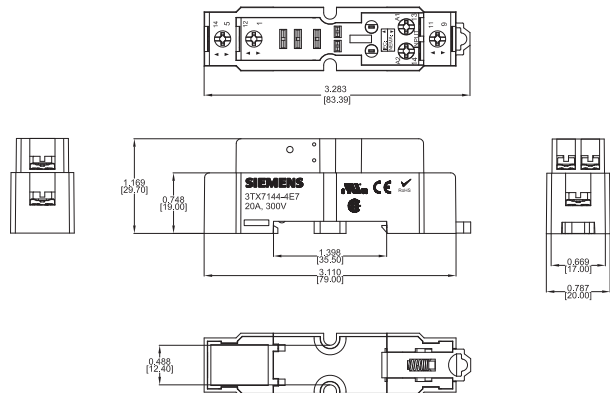
3TX7144-4E7
