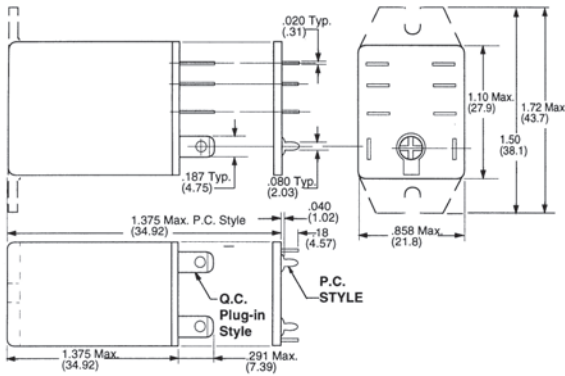
3TX7123
