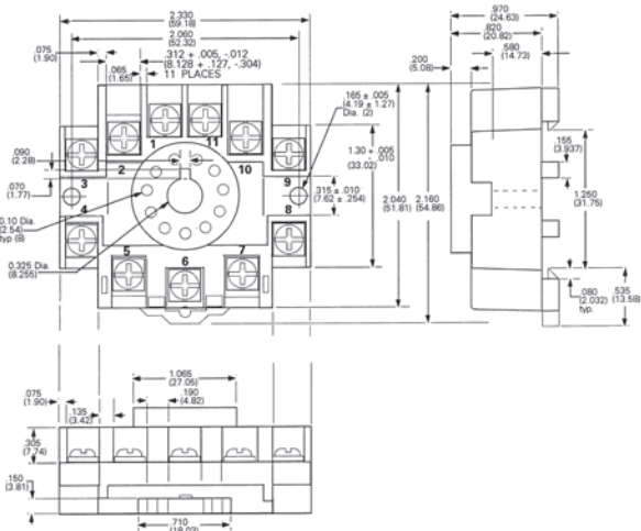
3TX7144-1E3
