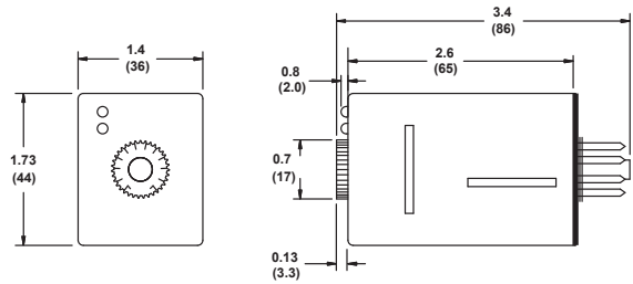
OND-DFOB (DPDT)
