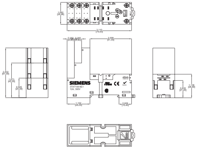
3TX7144-4E1
