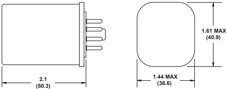
3TX7127 (DPDT)
