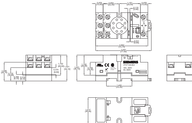
3TX7144-4E2
