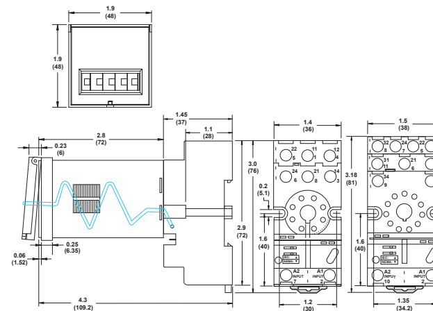
OND-DFPR-02 (DPDT)
