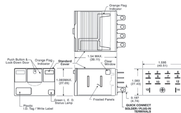
3TX7117 4PDT
