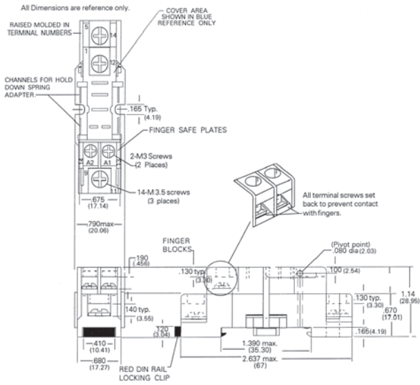
3TX7144-1E7
